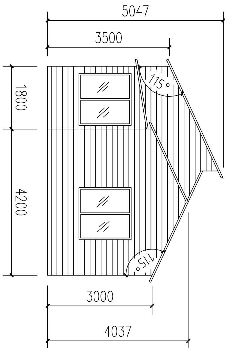
Right Elevation
