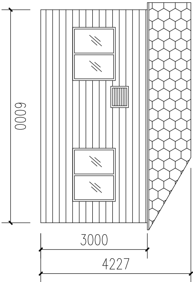
Right elevation
