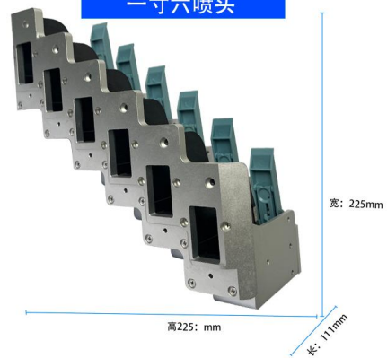
一寸六喷头
