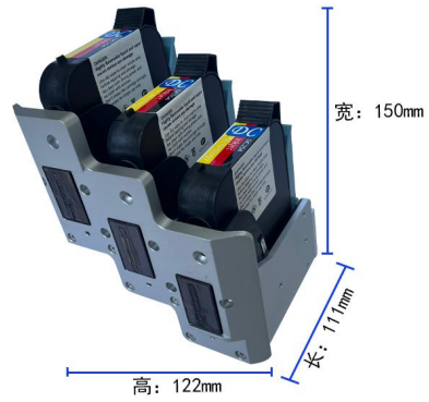
一寸六喷头
