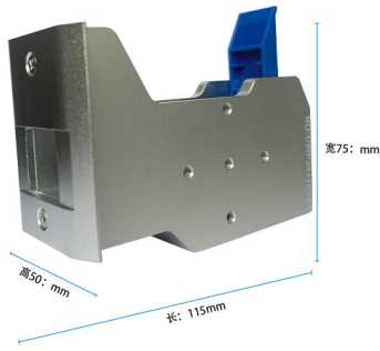
半寸双喷头
