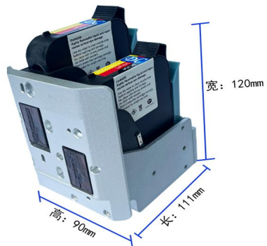
一寸三喷头
